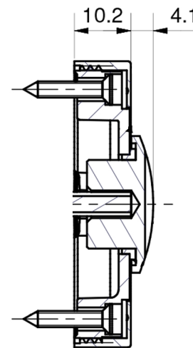
B-B ( 1 : 1 )
